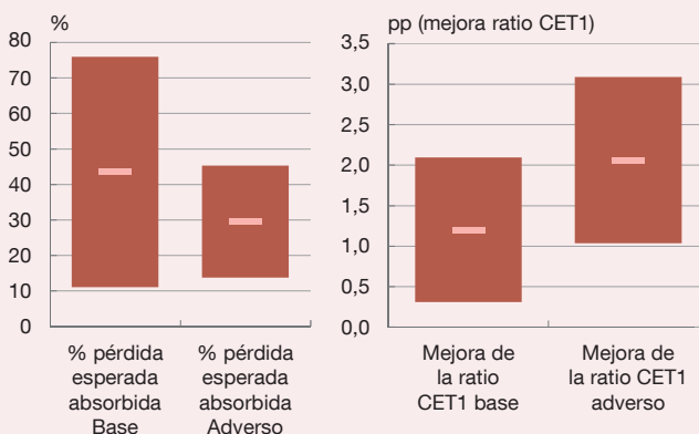
Gráfico 9 Efecto del programa de avales ICO (b) (c)
